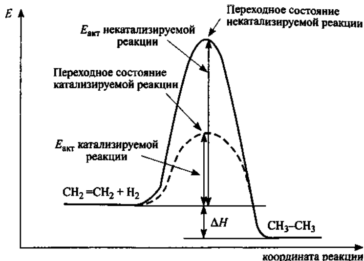
Рис. 10.1. Диаграмма потенциальной энергии в реакции гидрирования этилена без и в присутствии катализатора
