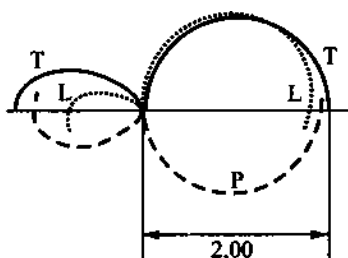
Рис. 1.11. Гибридные орбитали [10, с. 31]:
