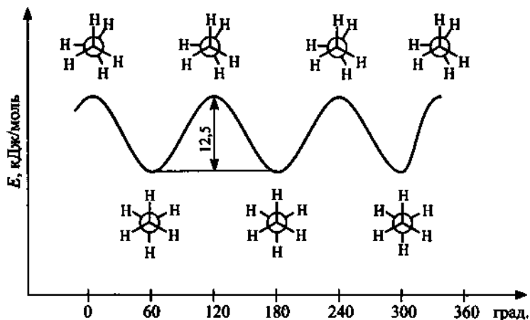
Рис. 3.3. Энергетический профиль вращения вокруг связи C-C этана
