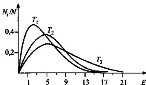
Рис. 4.2. Статистика Максвелла – Больцмана:
