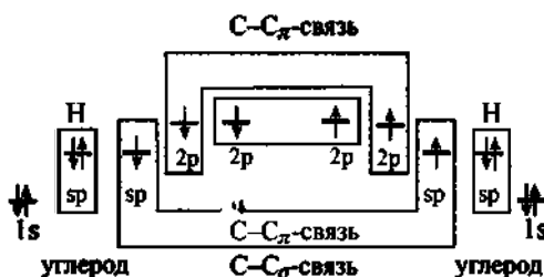
Образование связей в ацетилене
