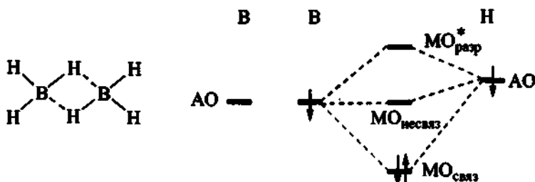
Рис. 1.7. Схема образования МО-орбиталей \text{B}_2\text{H}_6 (связи \text{B} \cdots \text{H-B} )
