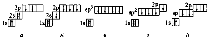
Рис. 1.10. Электронные конфигурации атома углерода:
