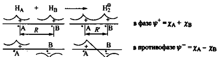
Рис. 1.2. Наложение атомных орбиталей в ионе H_2^+ :
