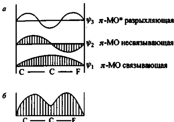
Рис. 2.4. Молекулярные орбитали фтористого винила: а — \pi -МО; б — суммарная р-, \pi -электронная плотность
