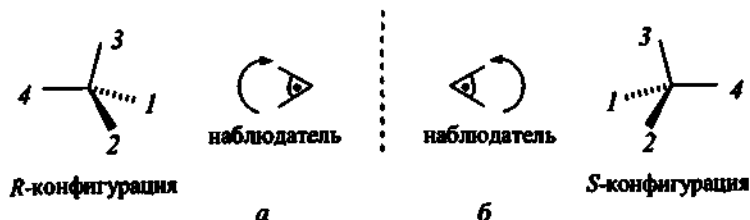
Рис. 3.2. Определение абсолютной конфигурации хирального центра 1 > 2 > 3 > 4 , где заместитель 4 — самый младший
