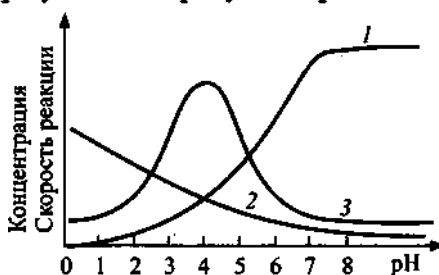
Рис. 19.1. Влияние pH на концентрации \text{CH}_3\text{C}(\text{OH})=\text{N}^+\text{H}_2 и \text{NH}_2\text{OH} , на скорость реакции образования оксима:
