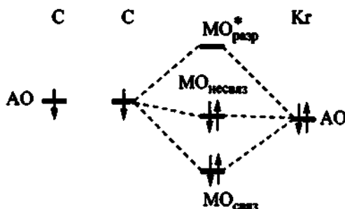
Рис. 1.6. Схема образования МО-орбиталей (\text{CF}_3)_2\text{Kf} (связи C-Kf)
